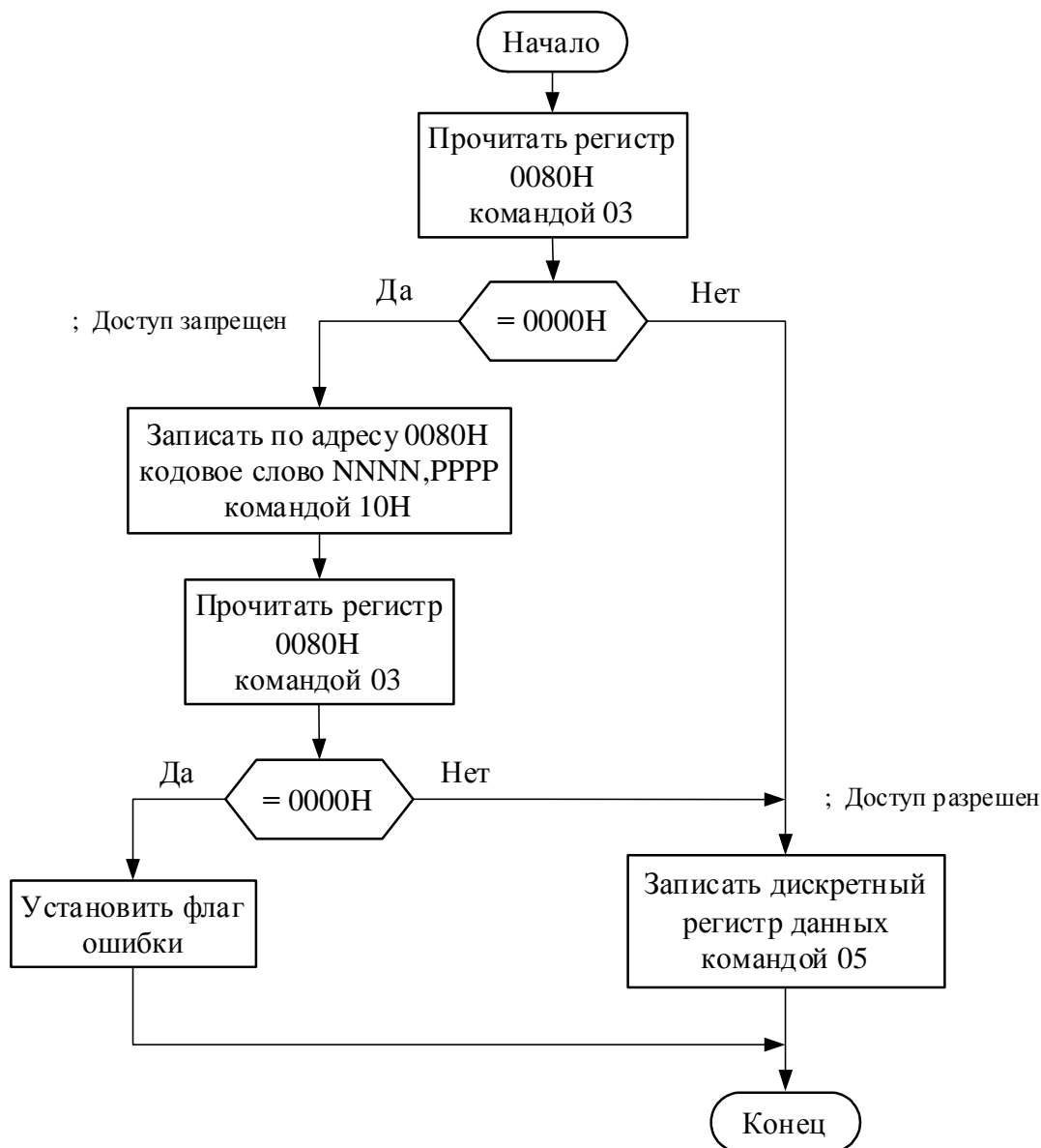
Рисунок 5 - Алгоритм управления записью в дискретные регистры данных модуля
